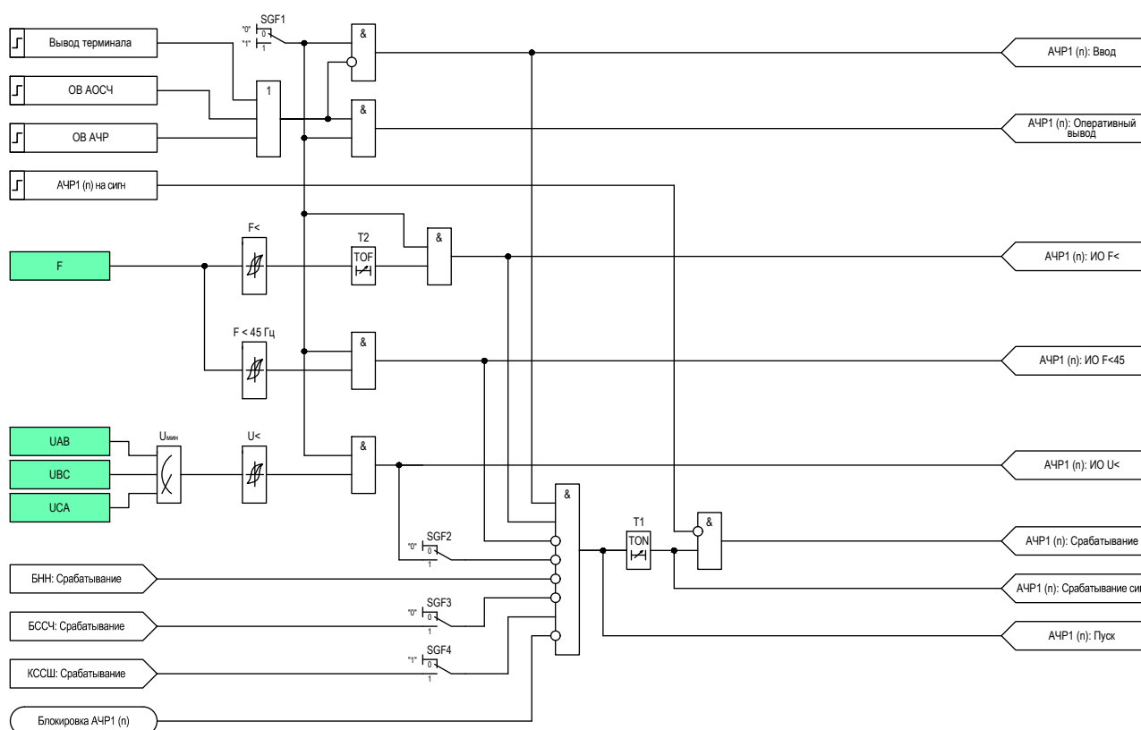
Рисунок 2.12 – Функциональная схема логики ступени АЧР
