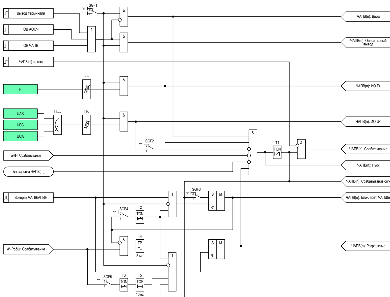
Рисунок 2.15 – Функциональная схема логики очереди ЧАПВ
