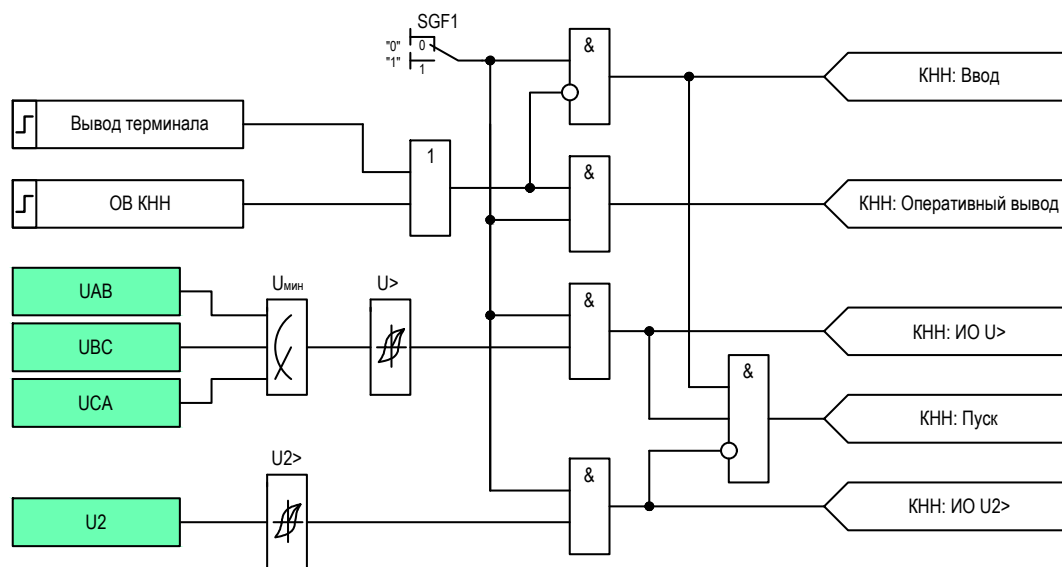
Рисунок 2.22 – Функциональная схема логики КНН
