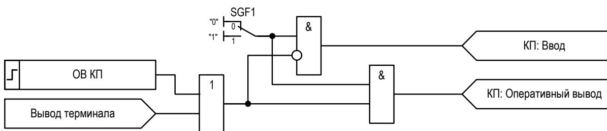
Рисунок 2.29 – Функциональная схема управления режимами работы КП
