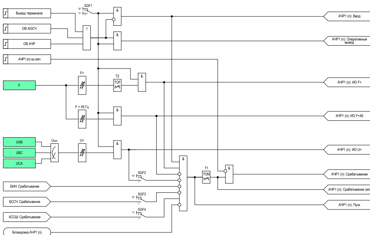
Рисунок 2.13 – Функциональная схема логики САЧР
