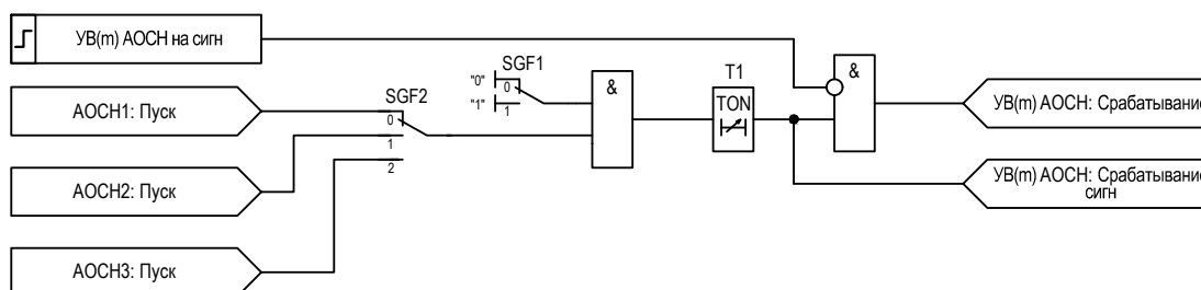
Рисунок 2.6 – Функциональная схема логики УВ АОСН
