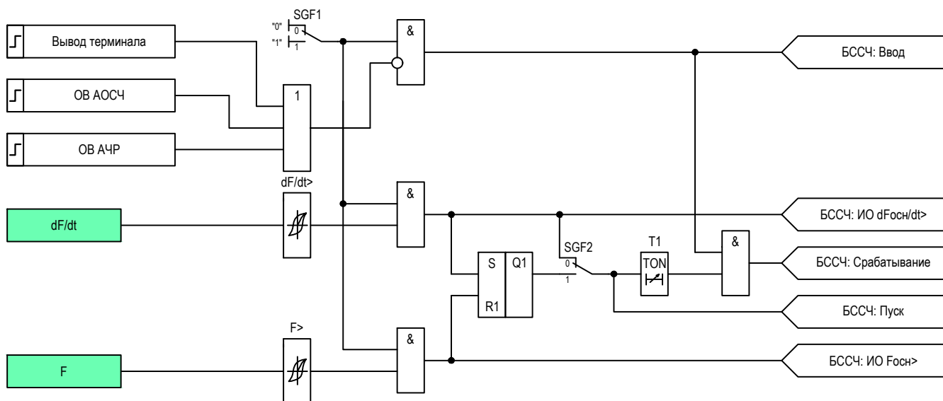
Рисунок 2.10 – Функциональная схема логики БССЧ
