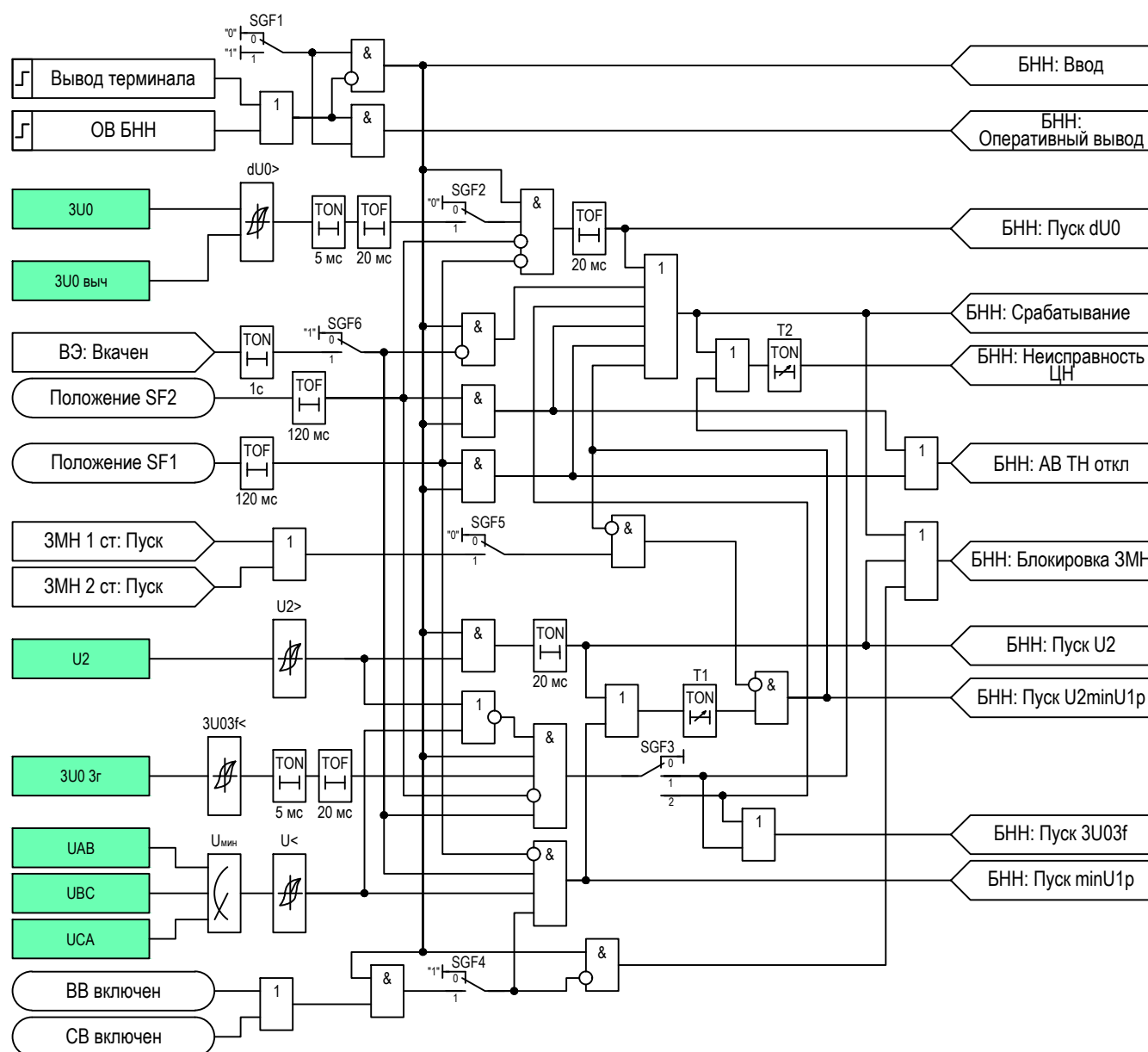
Рисунок 2.4 – Функциональная схема логики БНН
