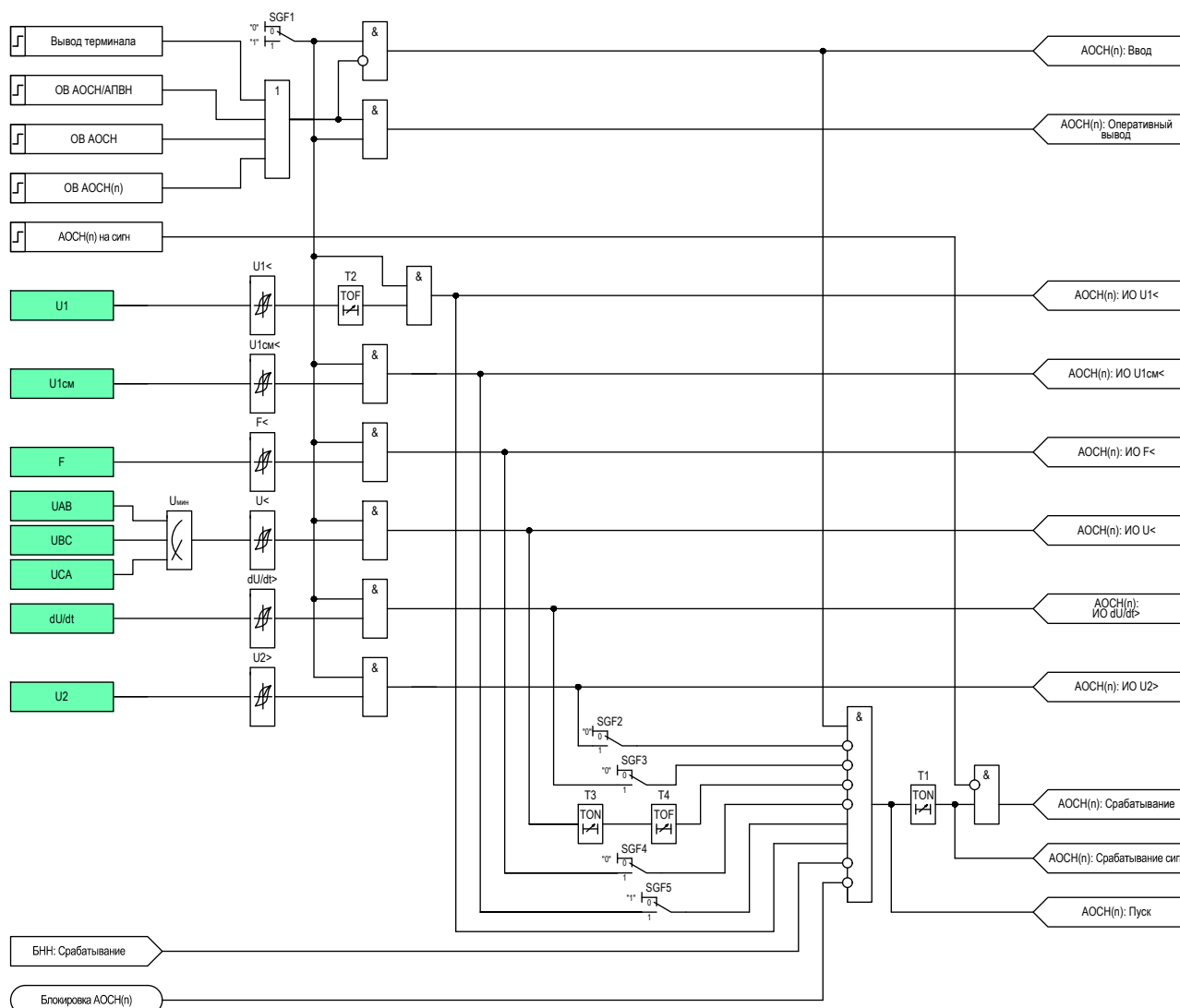
Рисунок 2.5 – Функциональная схема логики очереди АОСН
