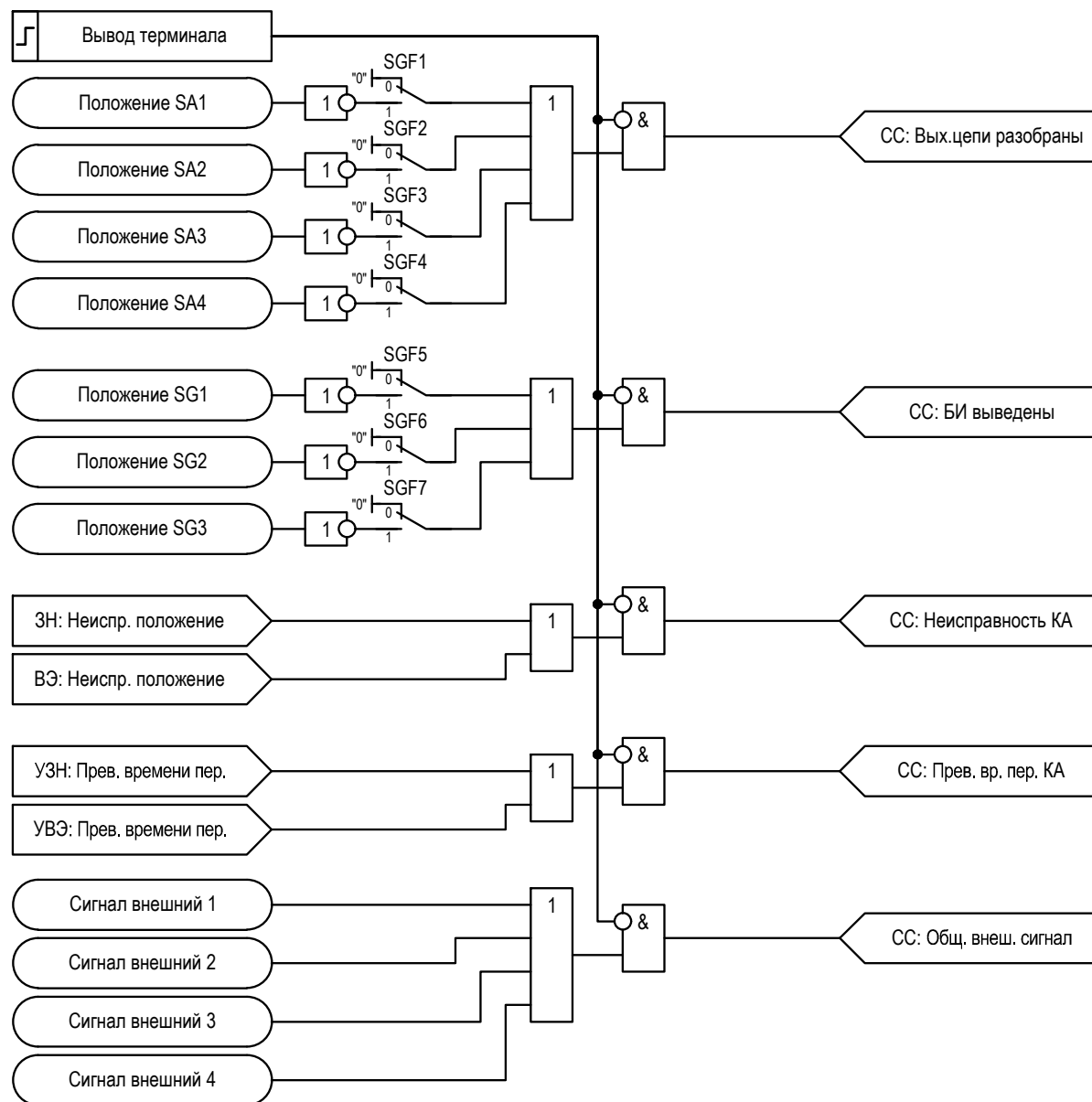
Рисунок 2.35 – Функциональная схема логики сборки сигналов
