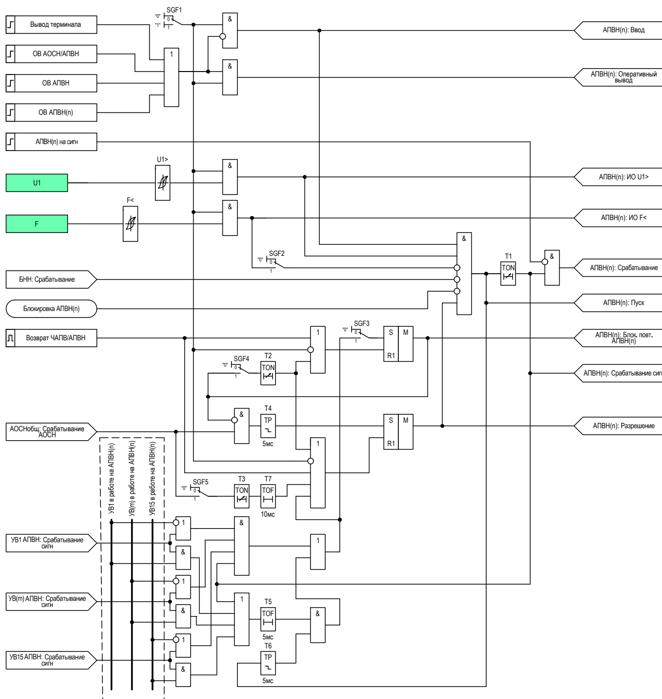
Рисунок 2.7 – Функциональная схема логики очереди АПВН
