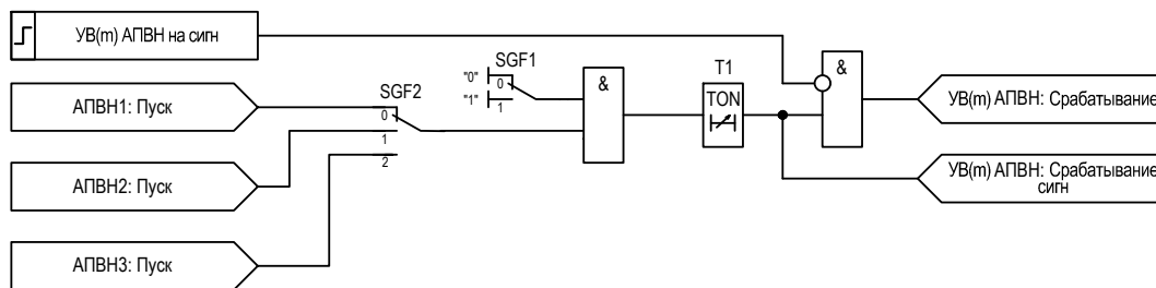
Рисунок 2.8 – Функциональная схема логики УВ АПВН
