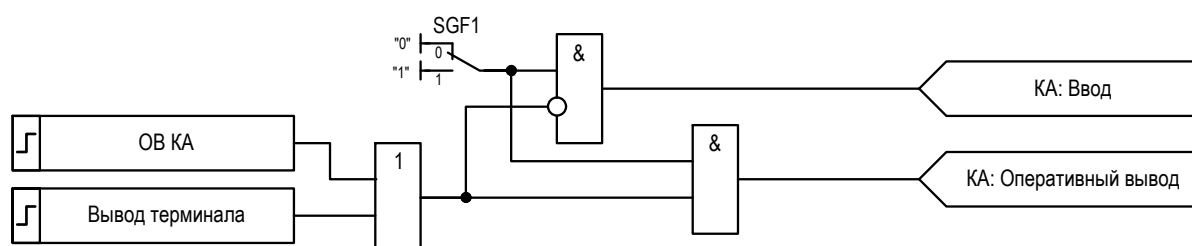
Рисунок 2.25 – Логика управления режимами КА
